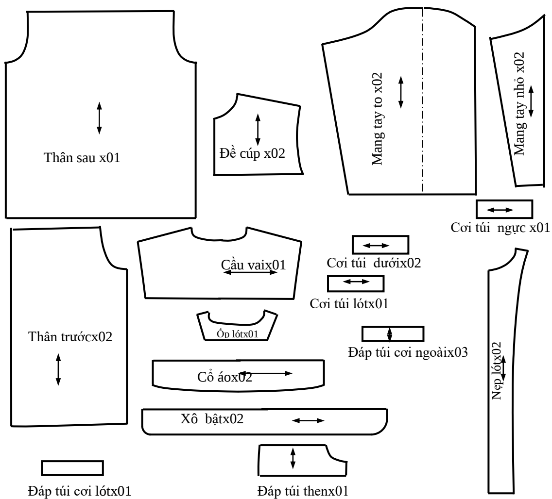
Hình 1-2. Các chi tiết lần chính áo Jacket 2 lớp gấu bông
